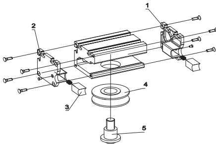
Zentrischer Bolzen
