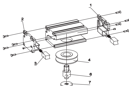
Boulon excentrique
