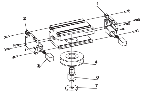
Exzentrischer Bolzen
