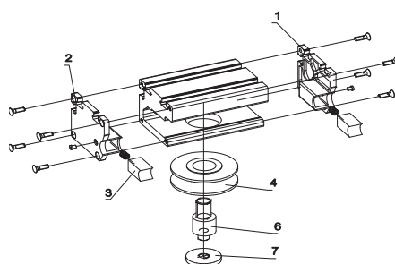
bulloni eccentrici
