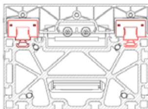
Kugelschienenführung
