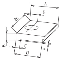
Befestigungslasche: Die Werte (in mm) für die Befestigung bitte der Tabelle entnehmen.
