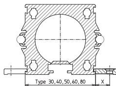
Befestigungslasche: Die Werte (in mm) für die Befestigung bitte der Tabelle entnehmen.
