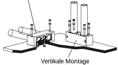
Vertikale Montage
