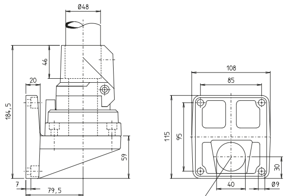
Kabeldurchführung
