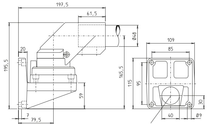
Kabeldurchführung
